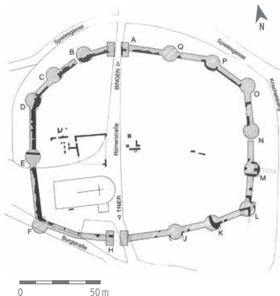
Plan der spätantiken Befestigung Neumagen.
