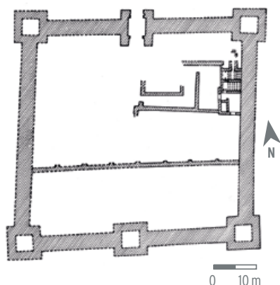
Schaan. Spät römisches Binnenkastell mit Innenbebauung und großem Magazin im Süddrittel.
