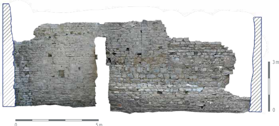
Koblenz. Blick von Norden auf die Außenschale der spätantiken Wehrmauer.
