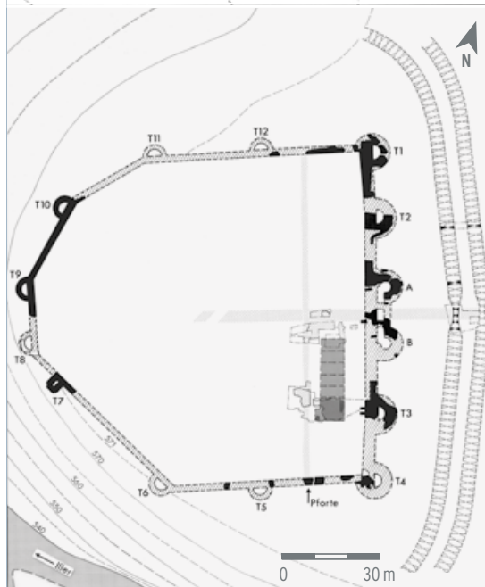
Kellmünz. Tetrarchisches Kastell mit Steinumwehrung, Abschnittsgraben und teilrekonstruierter Mannschaftsunterkunft um 300 n. Chr.
